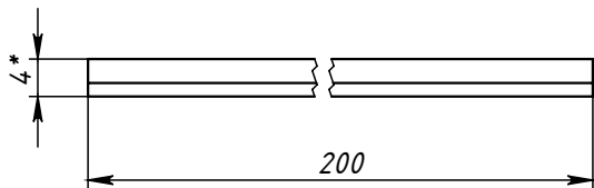
Поз.4 (Накладка) 1:1
